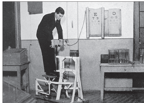
Általános munkabírás mérésére szolgáló készülék (Forrás: A BSzKRt tíz éve 1923–1933)
