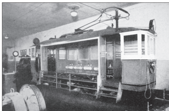
Metszetelt villamokocsi működő belső szerkezettel (Forrás: A BSzKRt tíz éve 1923–1933)
