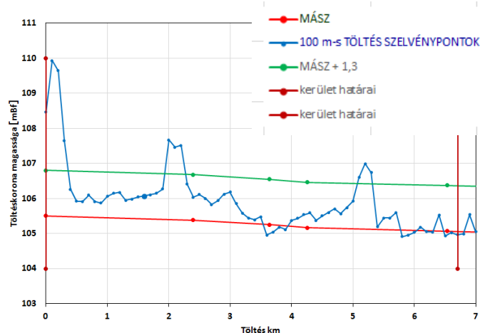
Vizsgálati területen a MÁSZ és MÁSZ +1,3m szintek és töltésmagasság
