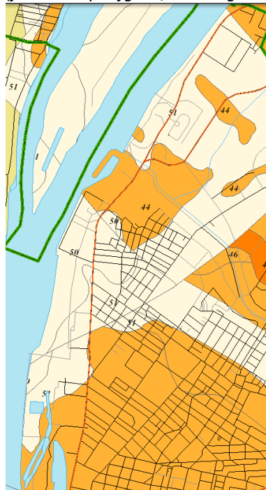
Fedetlen földtani térkép
