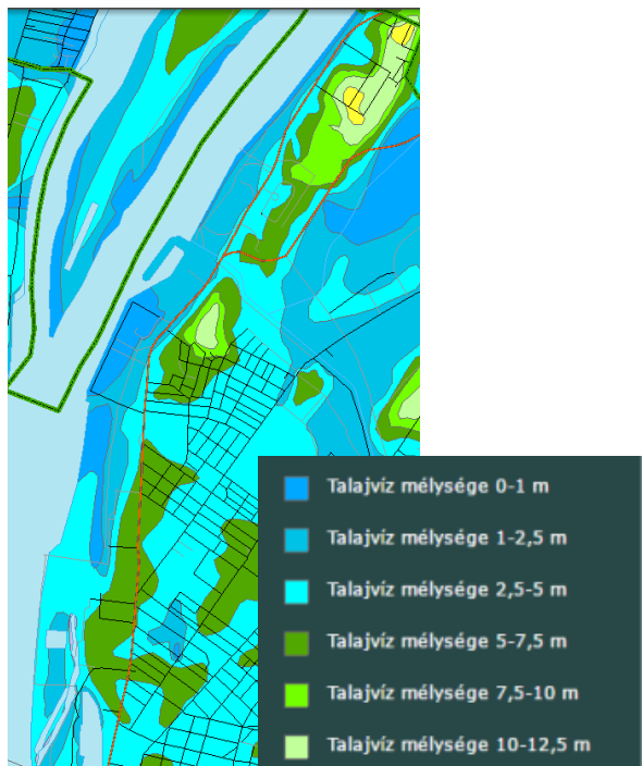
Talajvíz mélysége
