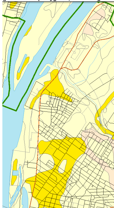
Felszíni földtani térkép
