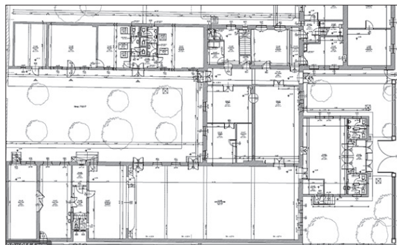
A katolikus kultúrház bontás előtti felmérési alaprajza (Forrás: Fusion Architekt Kft., Kissgergely Csaba)
