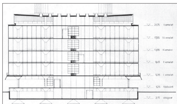
Az alagsorral és öt emelettel rendelkező épület metszete
