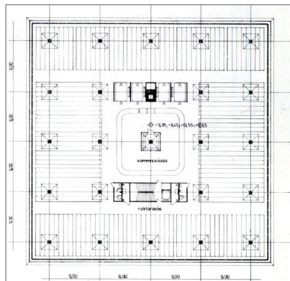
A raktárépület alaprajzán jól kivehetők a tartópillérek (A tervrajzok forrása: Magyar Építőművészet 1970/1. szám)
