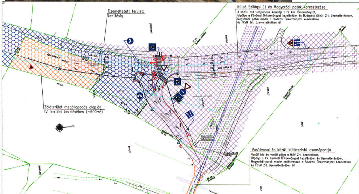
2. ábra Csomópont átépítés utáni állapot kezelői lehatárolási terv szerint
