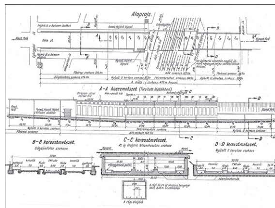
Az aluljáró alaprajza, hosszmetsete és keresztmetsetei
