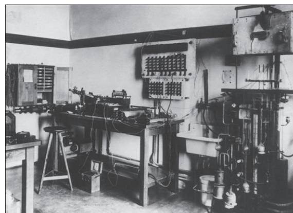
Egyesült Izzó, Elektroncső-laboratórium 1930 körül (Fotó: mek.oszk.hu)
