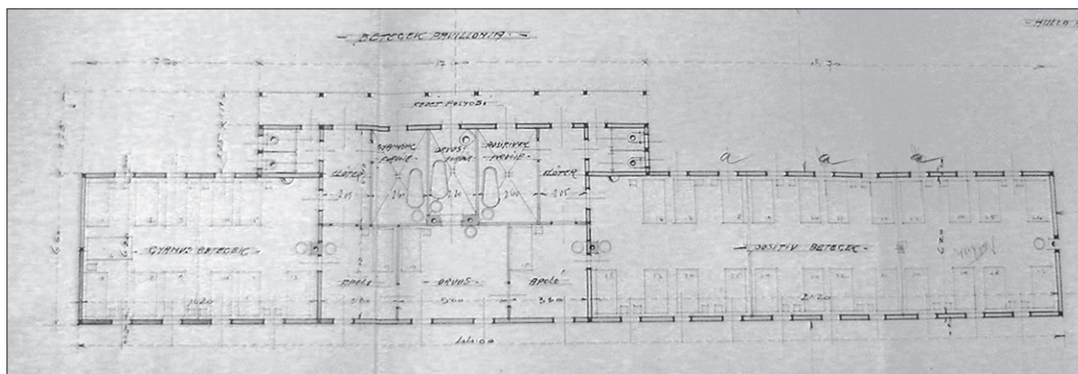
A járványkórház központi barakkjának tervrajza
