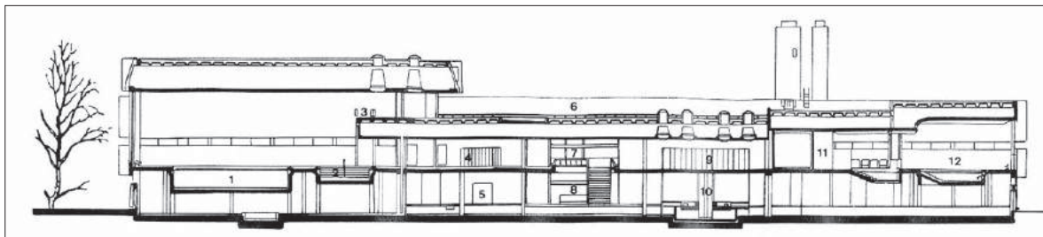
Az uszodaépület hosszmetsete
