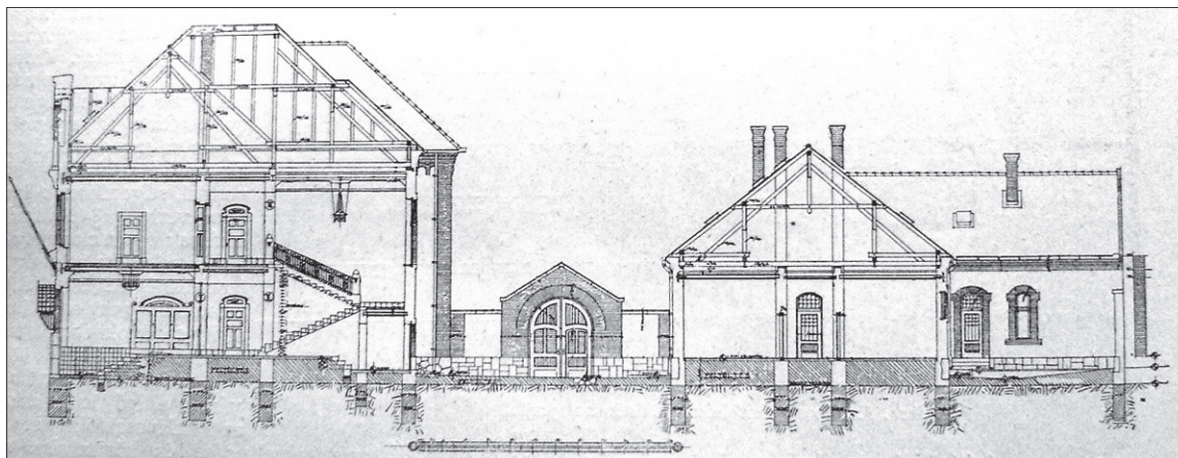
Az újpesti járásbíróház és fogdaépület metszete
