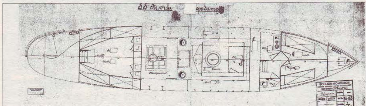
A Bácska (Baja) vontatógőzös alaprajza
