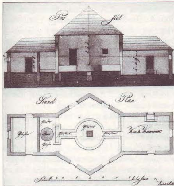
Káposztásmegyeri major, vízbízó és szecskavágó gép épületének terve (Magyar Országos Levéltár)
