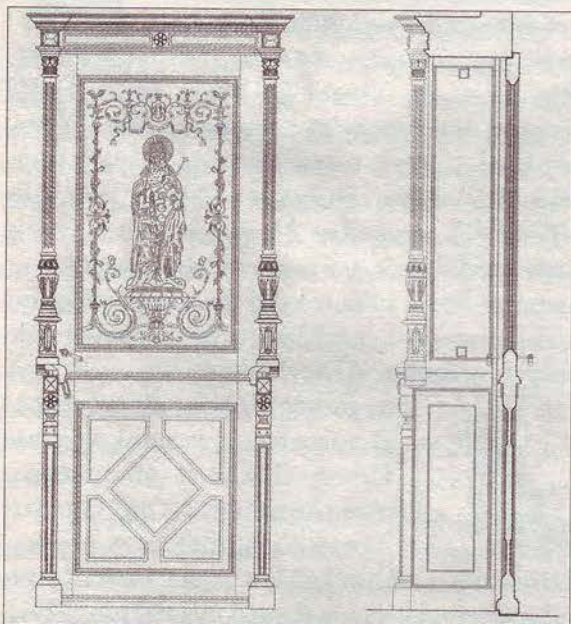
Az Árpád út 46. sz. alatti patika belső ajtaja (feldolgozta: Székely György építészhallgató – 1999)
