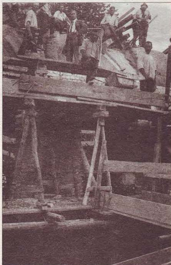
Az aggok háza bővítése – új szint ráépítése dongaboltozatos lefedéssel
